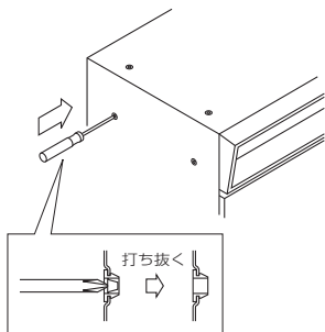
■ 図A〈連結穴のあけ方〉
