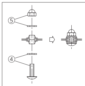
■ 図B〈連結部詳細〉
